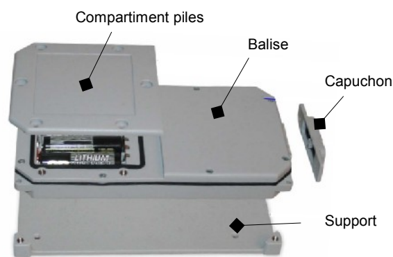
Vue éclatée
